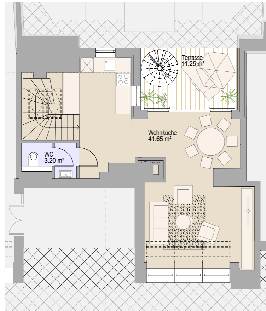
2. DACHGESCHOSS
